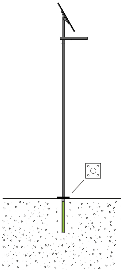
GRONDPLAAT
