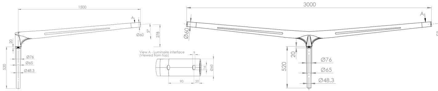
DIO TOP SIMPLE S1500 / Pole Ø76
